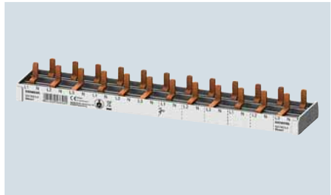
Штыревая сборная шина для компактных устройств 5SV1/5SV6/5S..0
