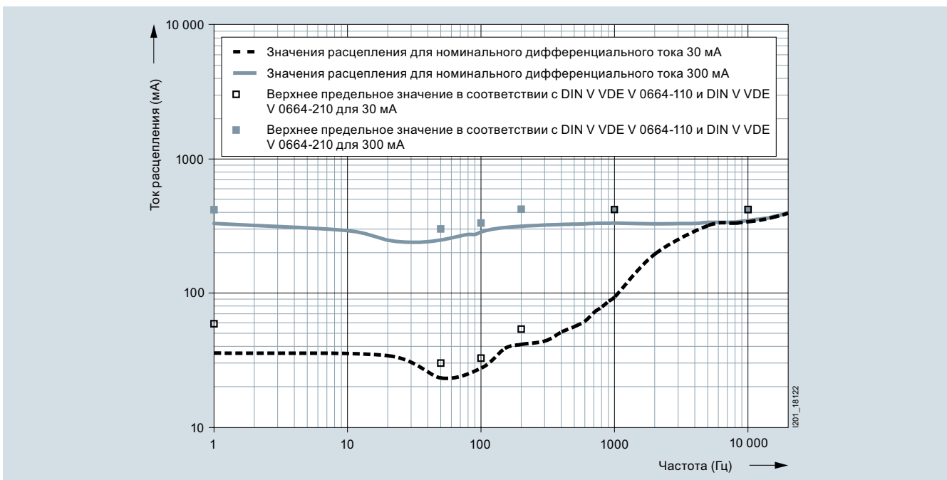
Зависимость тока расщепления от частоты для устройств типа В+
