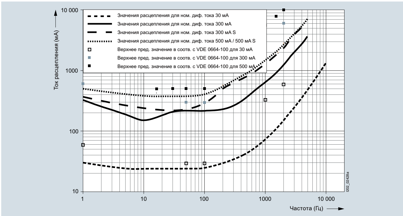
Зависимость тока расщепления от частоты для устройств типа В
