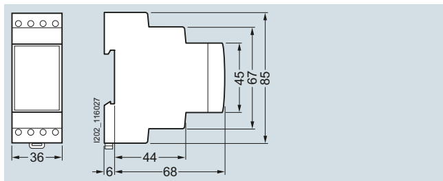
RCM аналоговое, 5SV8000-6KK
