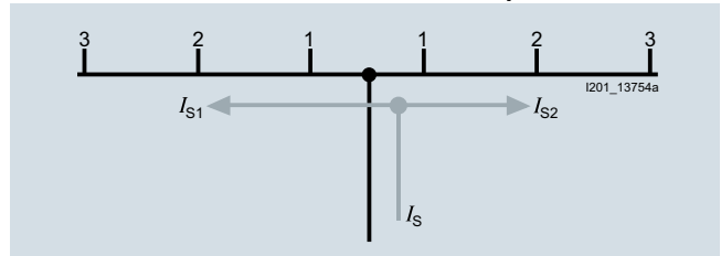
Ввод питания вдоль шины или в середине
