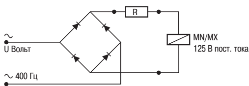
Схема подключения
