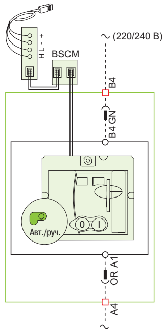
Коммутационный мотор-редуктор (MTc)
