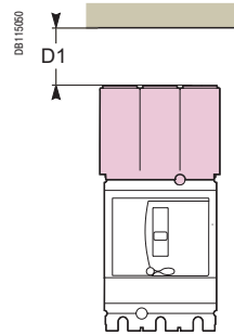
Аппараты с разделителями полюсов или длинной клеммной заглушкой
