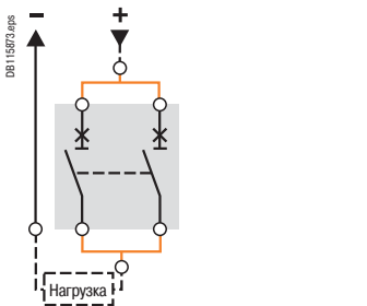
Выбор 3: 2-полюсный Compact NSX100N DC с параллельным подключением полюсов
