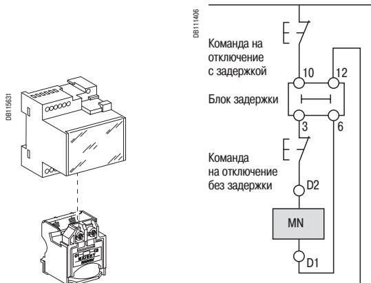
Электромонтажная схема аварийного отключения с расцепителем MN и блоком задержки
