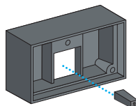
Тамбур и удлинитель для рычага управления, обеспечивающие IP4 в положениях «вквачено» и «выкачено»
