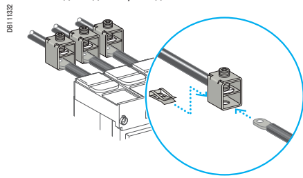
Присоединение кабелей без наконечников к NSX100 - 250
