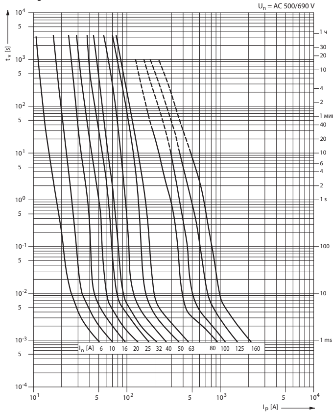
Времятоковая характеристика P51R06 gR, aR
