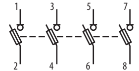
FH000-1.. + FH000-3..
