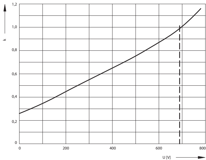
Коэффициент „k“ зависимости I^2t_c от рабочего напряжения (I^2t_c)_{(U)} = k \times I^2t_c
