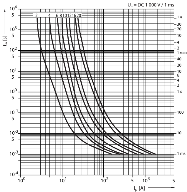
Времятоковая характеристика PC10 gPV
