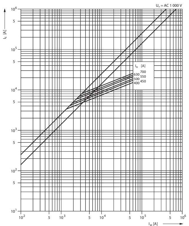
Характеристика токоограничения P50U10, P50V10 aR
