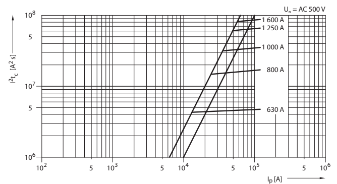
Характеристика I^2t_c PN4a gG
