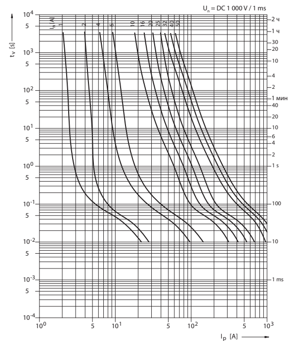
Времятоковая характеристика PT22
