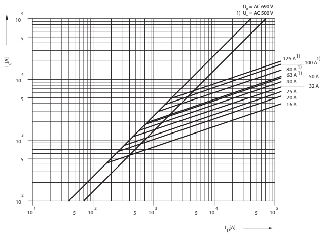
Характеристика токоограничения PV22 gG
