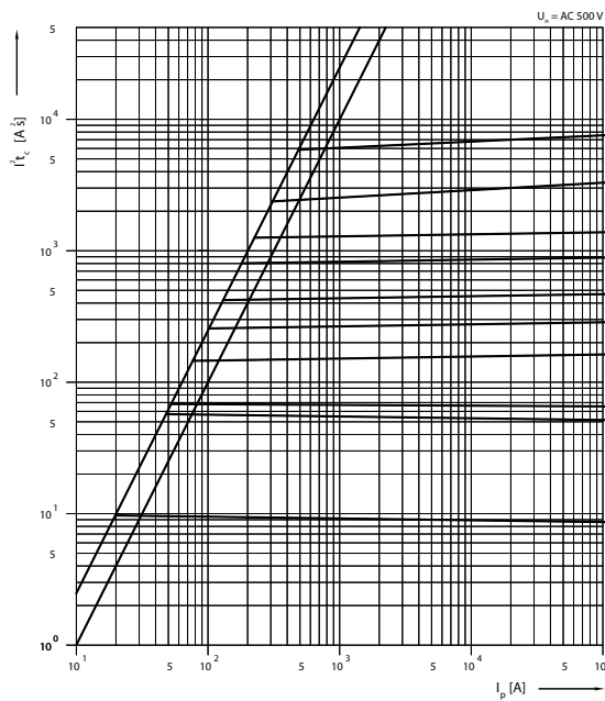
Характеристика I 2 t c PVA10, PV10 1) gG
