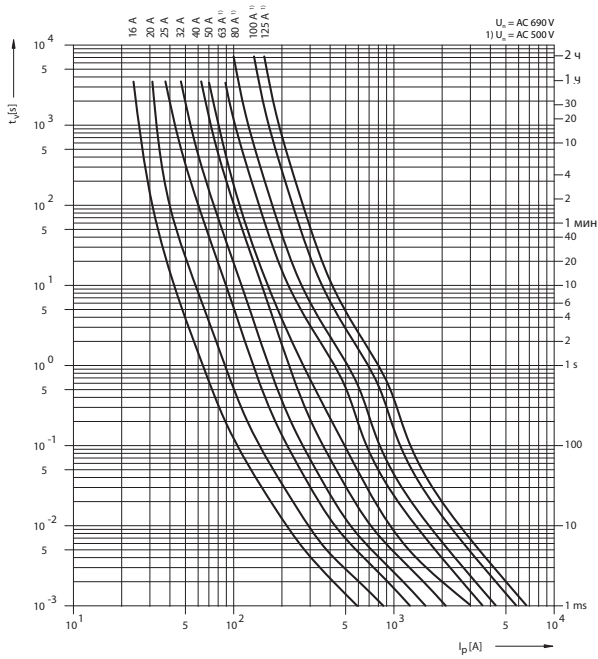
Времятоковая характеристика PV22 gG
