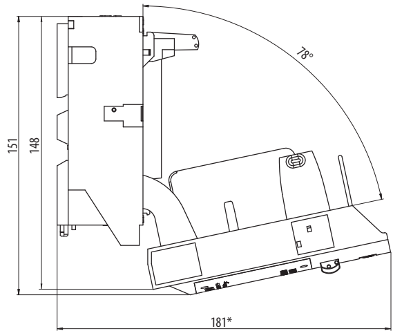
FH000-3A/T, FH000-1A/T и FH000-3L/T
