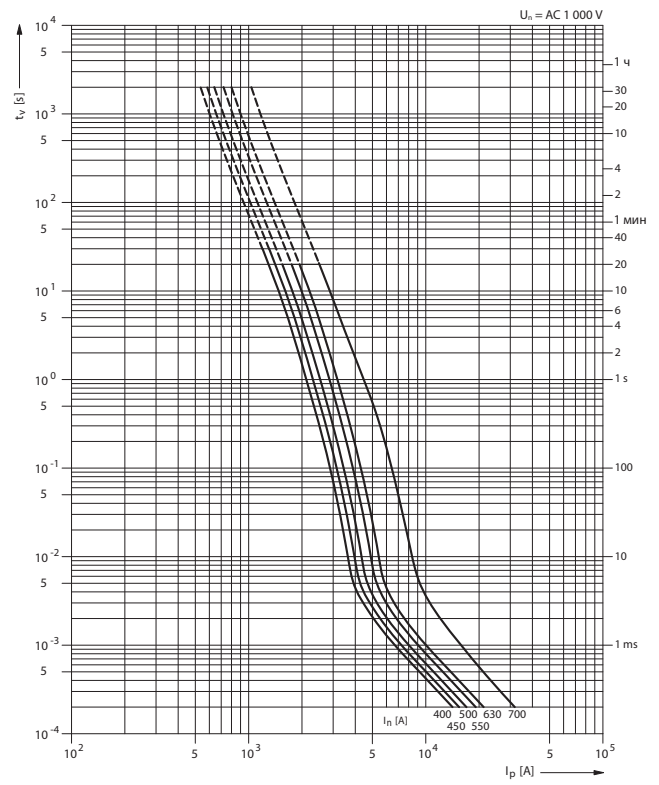
Времятоковая характеристика P50U10, P50V10 aR
