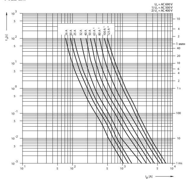
Времятоковая характеристика PV22 aM
