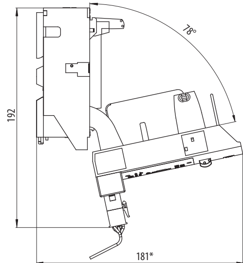
FH000-3S/T и FH000-1S/T
