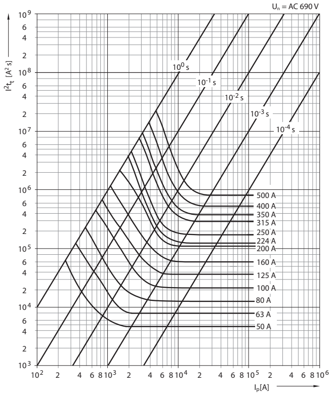
Характеристика I^2t PHNA1, 2, 3 gG
