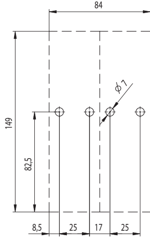
2-полюсный разъединитель
