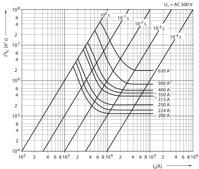
Характеристика I^2t PNA3, PN3 1) gG
