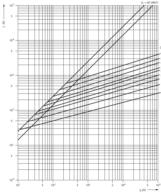
Характеристика токоограничения PV514 gR, aR
