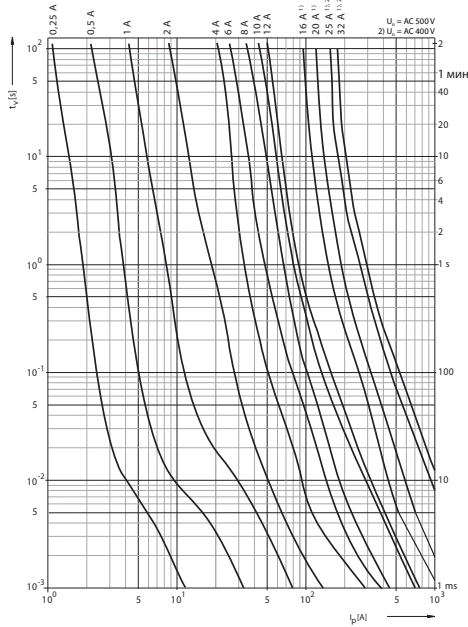
Времятоковая характеристика PVA10, PV10 1) aM
