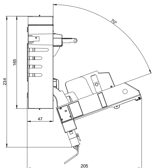
FH00-3S/F и FH00-1S/F
