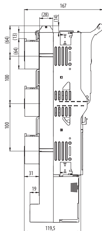
FSD00-33K-FC - M...
