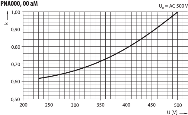
Коэффициент „k“ зависимости I^2t_c от рабочего напряжения (I^2t_c)_{(U)} = k \times I^2t_c
