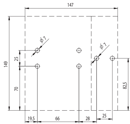
3-полюсный и 4-полюсный разъединитель
