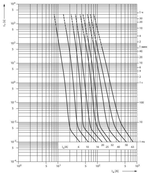
Времятоковая характеристика для PV514 в OPVP14
