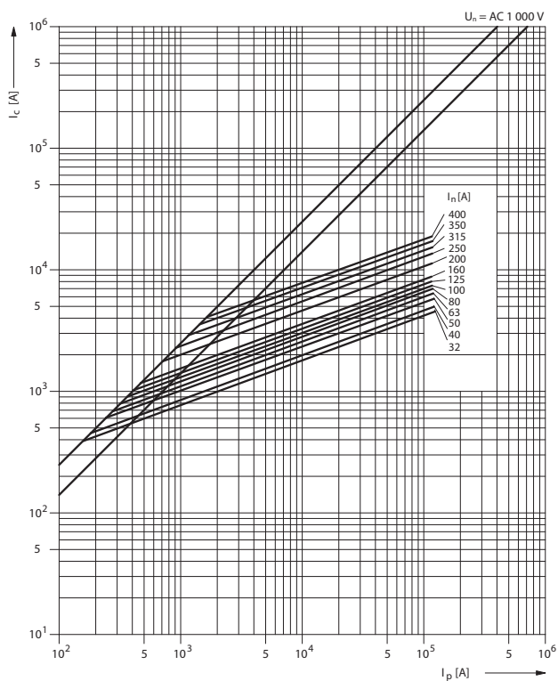
Характеристика токоограничения P40U10 gR, aR
