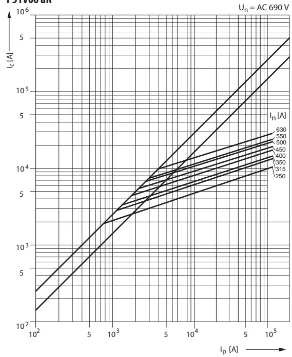
Характеристика токоограничения P51V06 aR
