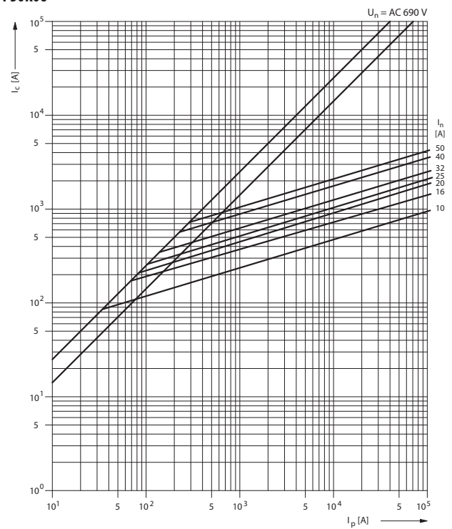
Характеристика токоограничения P50K06
