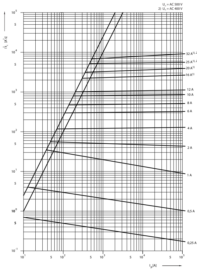
Характеристика I^2t_c PVA10, PV10 1) aM
