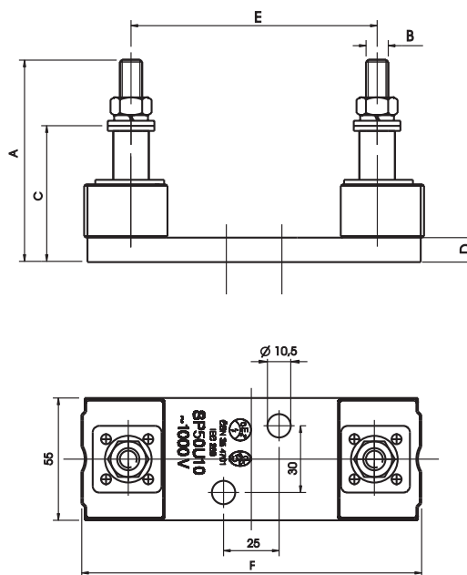
SP50.10, SP50X16
