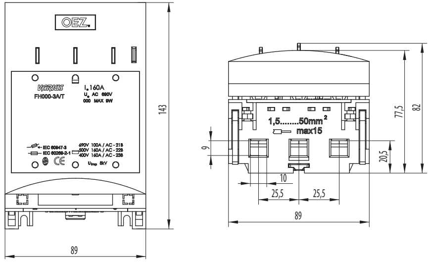
FH000-3A/T и FH000-3L/T
