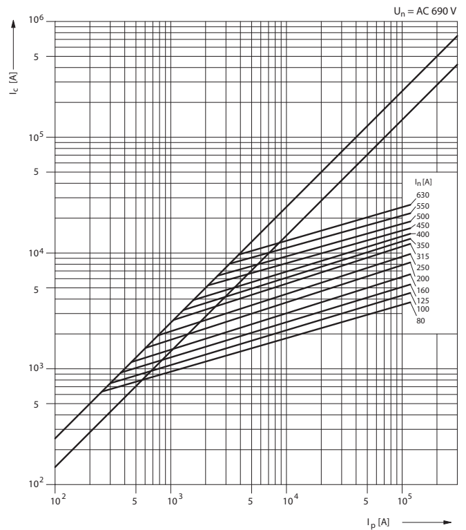
Характеристика токоограничения P50U06, P52U06 aR
