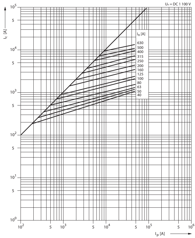
Характеристика токоограничения P50V16 gR, aR
