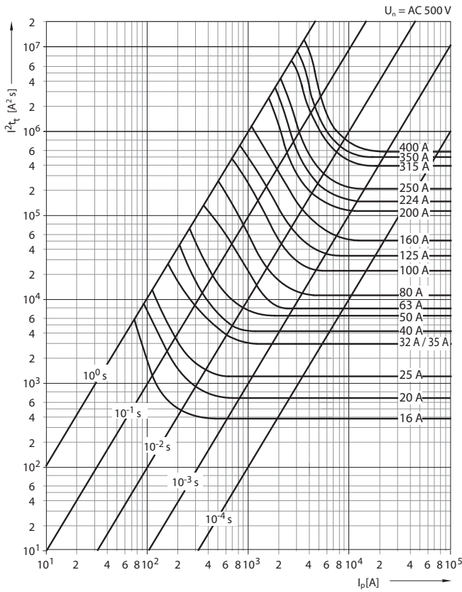
Характеристика I^2t PNA1, 2 gG
