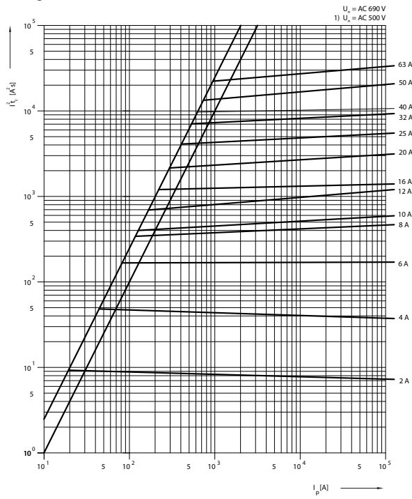
Характеристика I^2t_c PV14 gG
