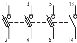
FH000-1.. + FH000-3..
