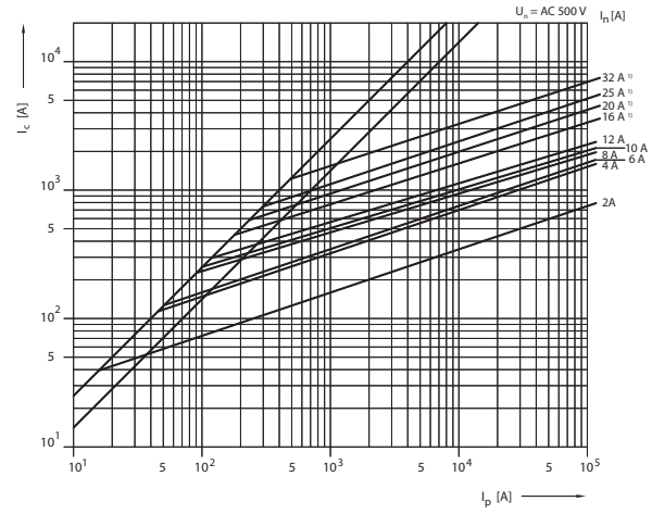
Характеристика токоограничения PVA10, PV10 1) gG
