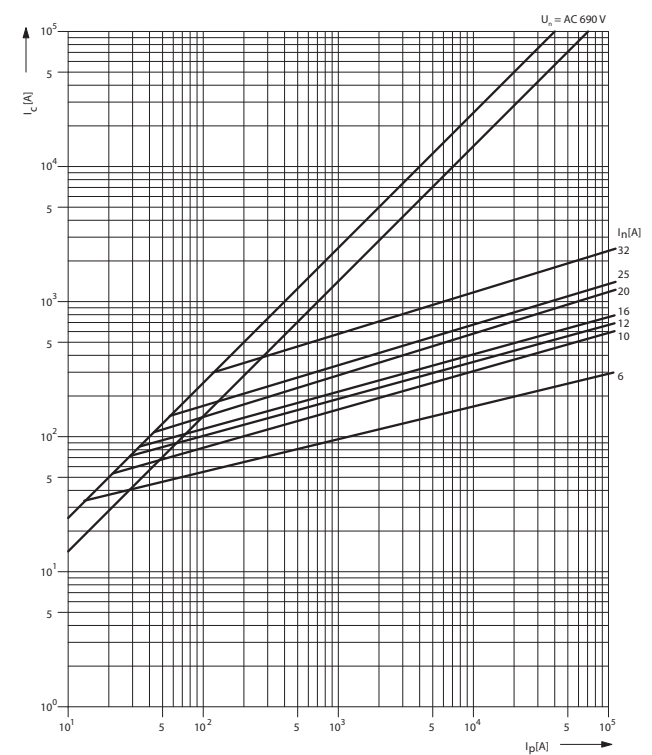
Характеристика токоограничения PV510 gR
