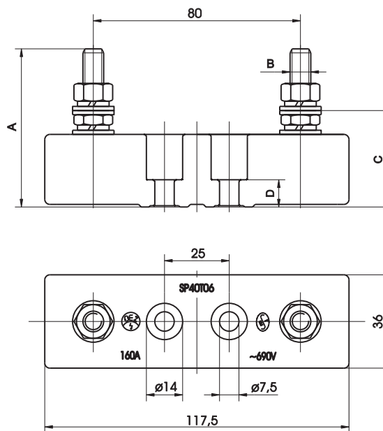
SP40T06, SP41T06
