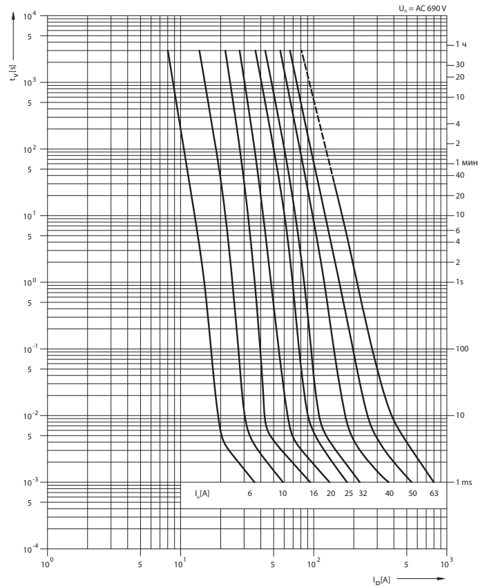
Характеристика токоограничения PV510 gR
