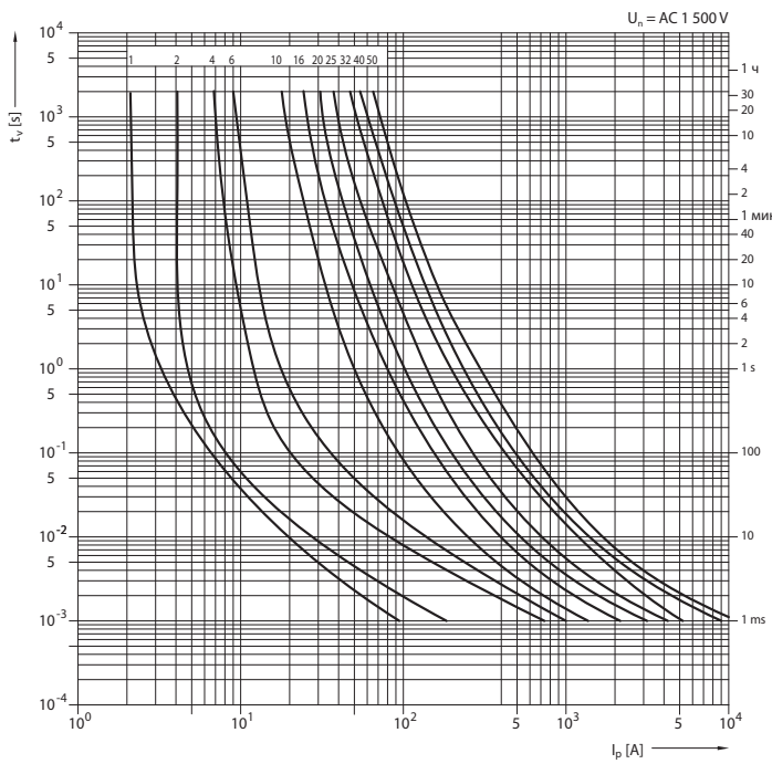
Времятоковая характеристика PT22
