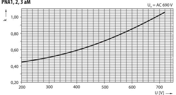
Коэффициент „k“ зависимости I^2t_c от рабочего напряжения (I^2t_c)_{(U)} = k \times I^2t_c
