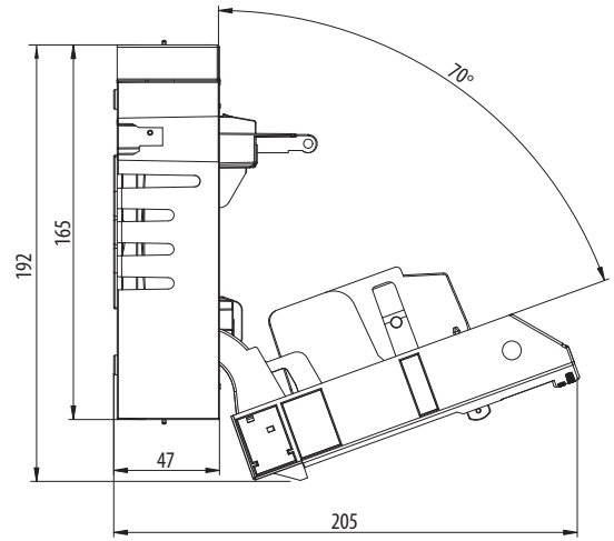
FH00-3S/F и FH00-1S/F
