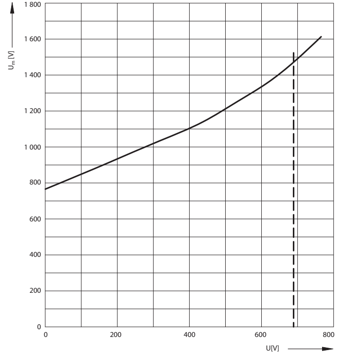
Зависимость перенапряжения от рабочего напряжения
