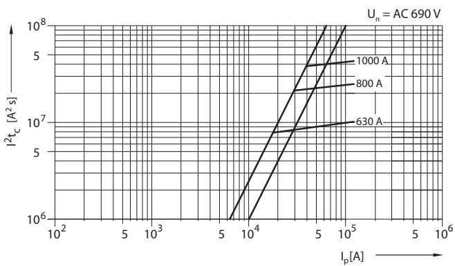
Характеристика I^2t_c PHN4a gG
