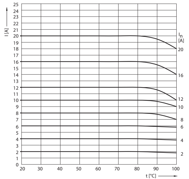
Влияние температуры окружающей среды PC10 gPV
