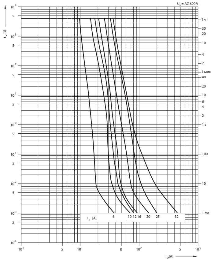
Времятоковая характеристика PV522 gR, aR
