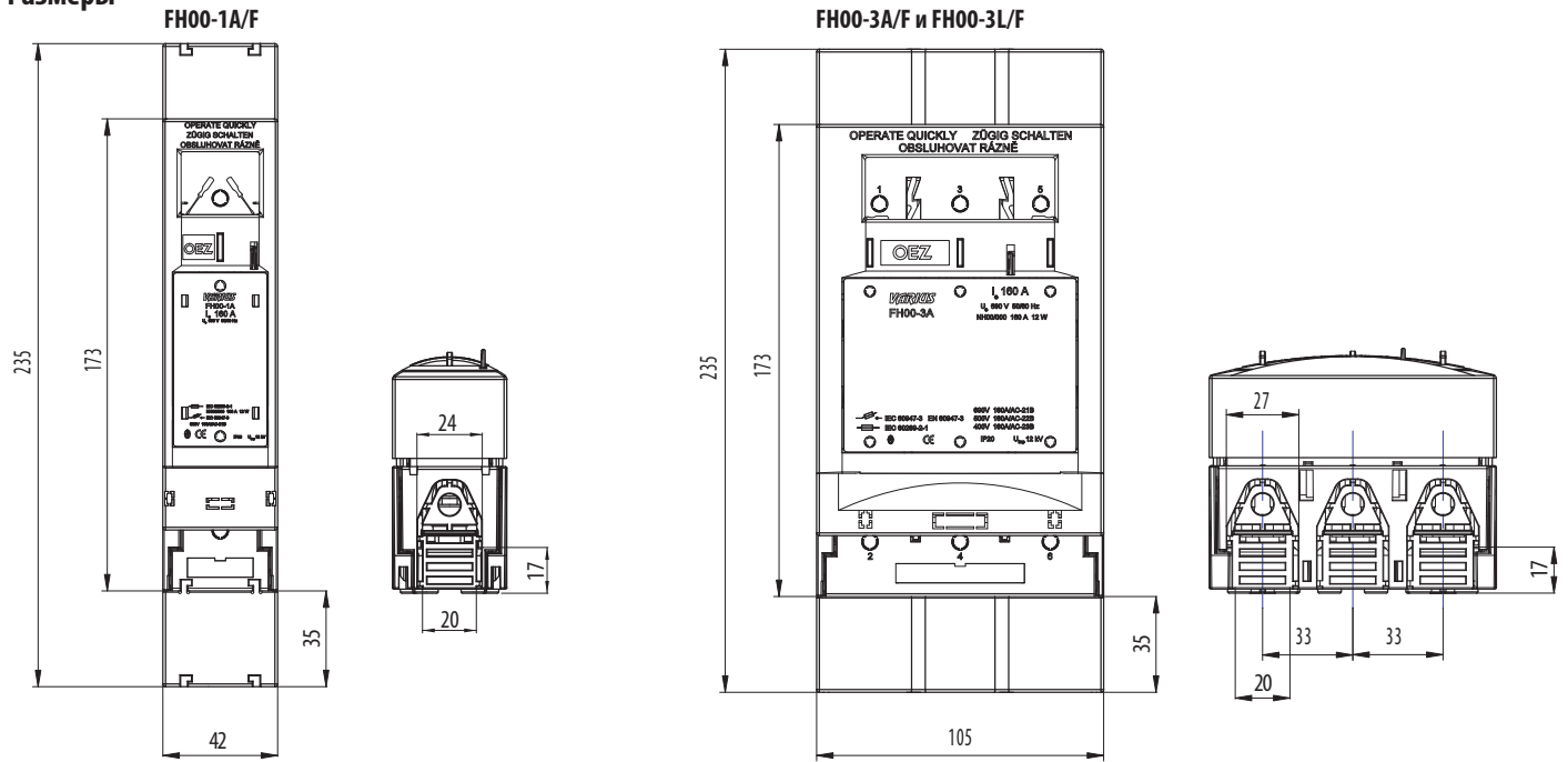
FH00-1A/F, FH00-3A/F и FH00-3L/F
