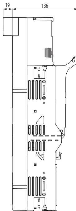
FSD00-33K-FC кабельный вывод сверху
