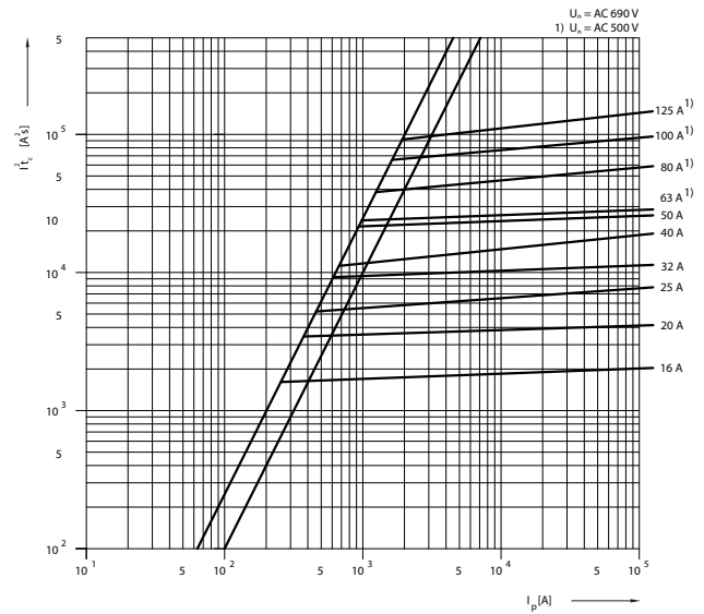
Характеристика I^2t_c PV22 gG
