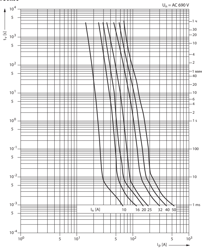
Времятоковая характеристика P50K06
