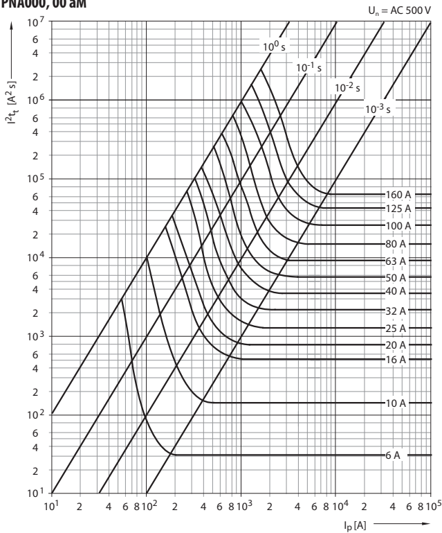
Характеристика I^2t_c PNA1, 2, 3 aM
