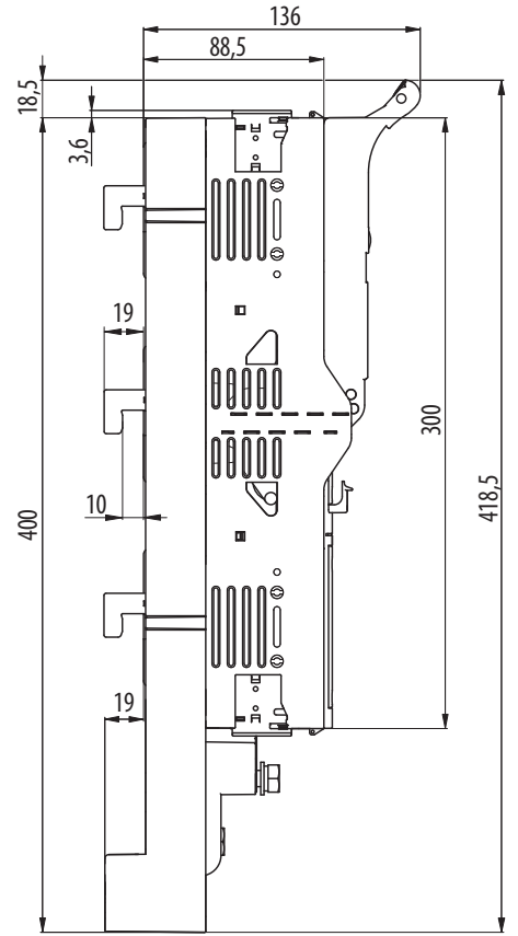
FSD00-33K-F + CS-F500-3H
