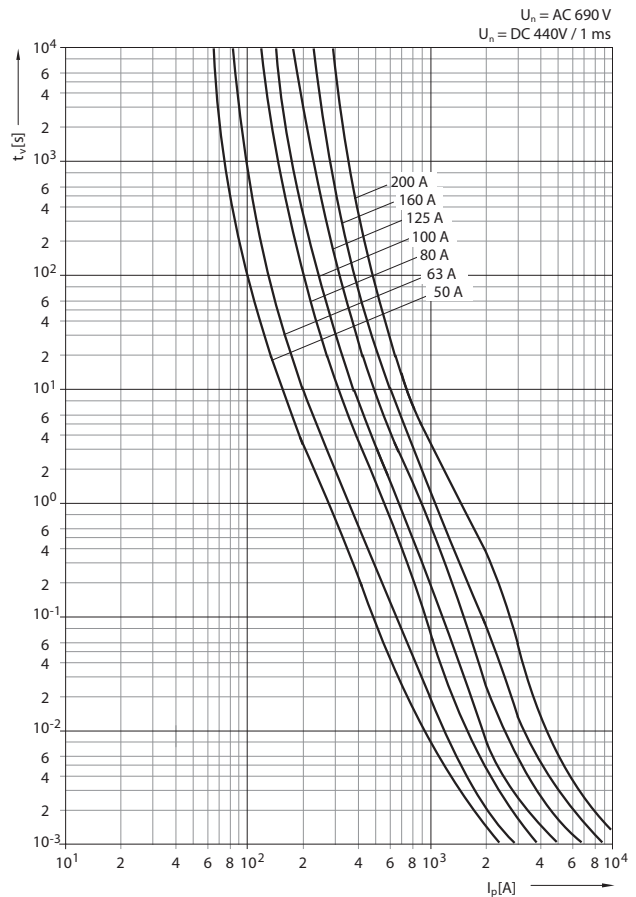
Времятоковая характеристика PHNA1 gG
