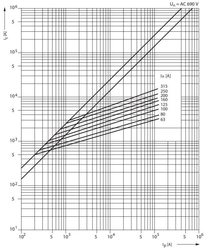
Характеристика токоограничения P51U06 gR, aR
