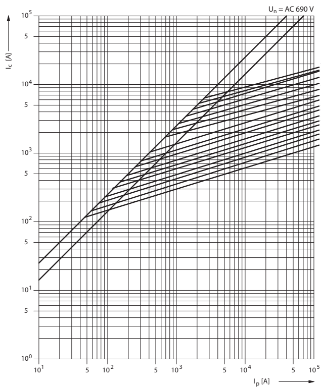
Характеристика токоограничения P50T06 gR, aR
