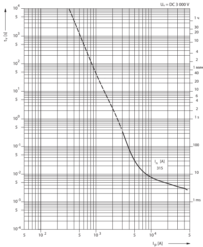
Времятоковая характеристика P50V30
