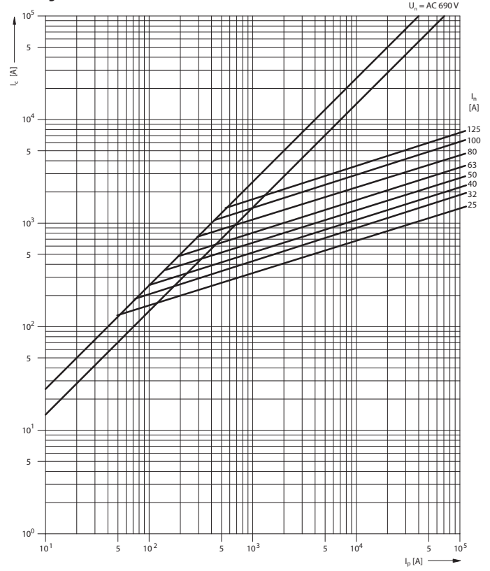
Характеристика токоограничения PV522 gR, aR
