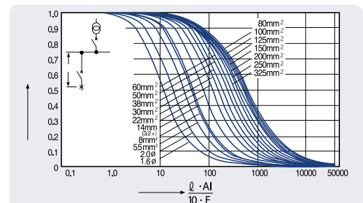
Рис. 12. Понижающий коэффициент b для кабеля (600V IV)
