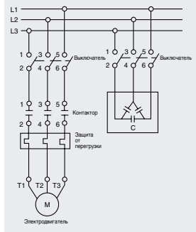
Стандартная схема подключения
